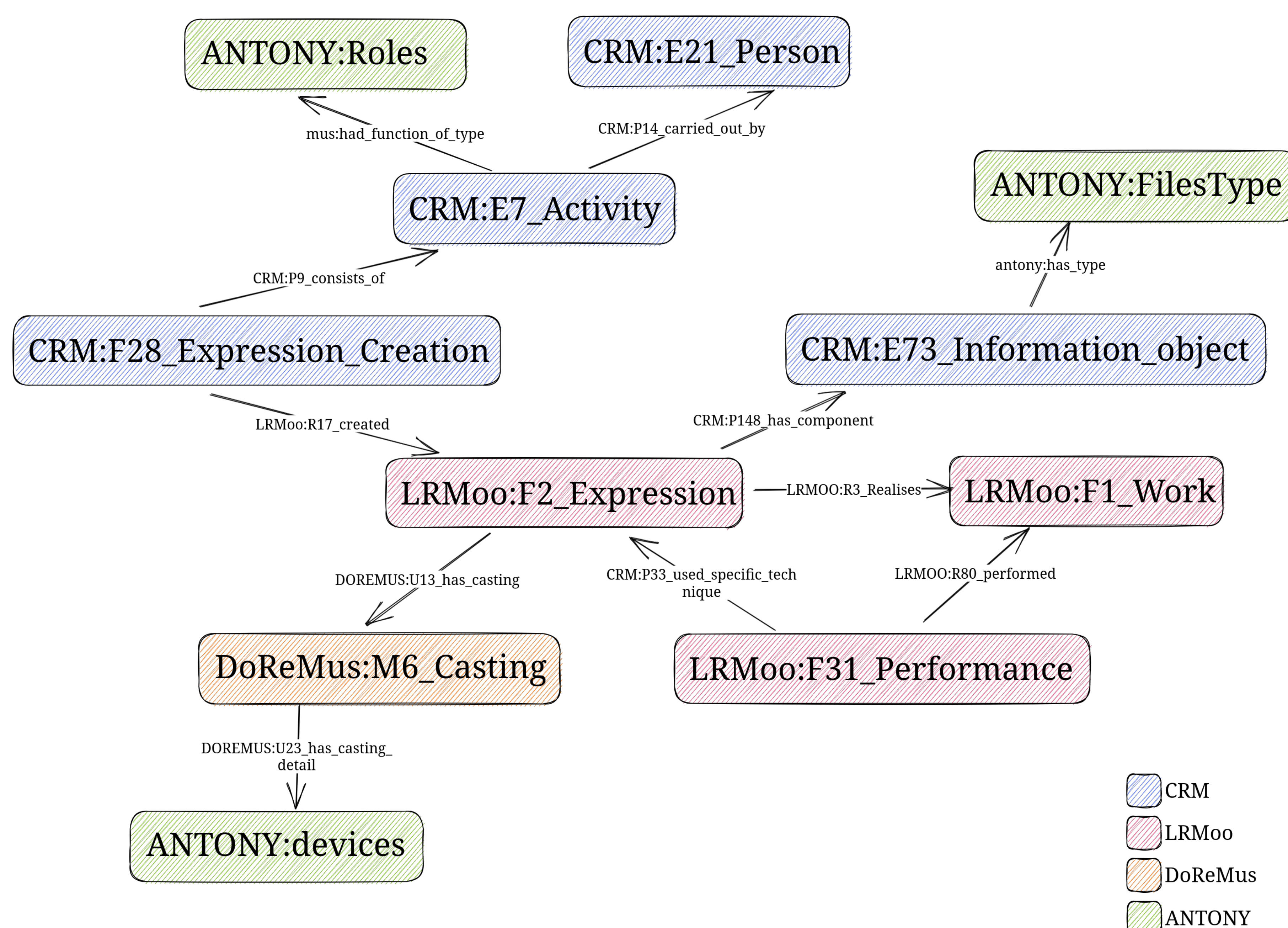
Modèle de données RDF de l'application ANTONY
